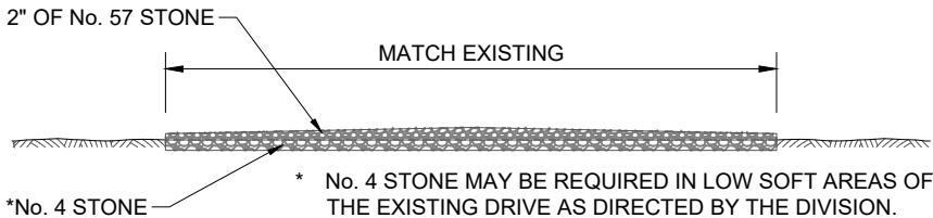
SECTION A-A'
